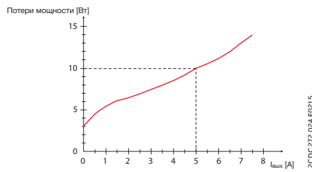
График зависимости средних потерь мощности (тепловыделения) от выходного тока
