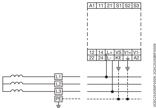
3-проводная сеть переменного тока
