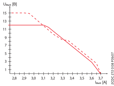
CP-E 12/2.5
