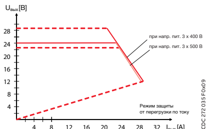
CP-T 24/20.0 Режим прерывания питания (hiccup mode) при перегрузке
