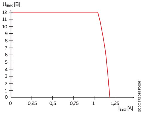
CP-D 12/0.83
