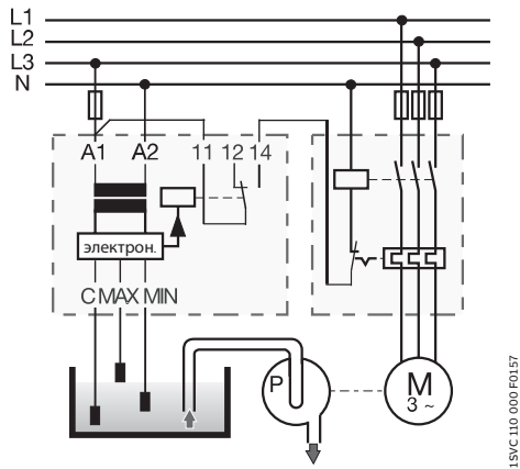
Контроль уровня жидкости — слив
