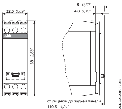
Пломбируемая прозрачная крышка COV.11
