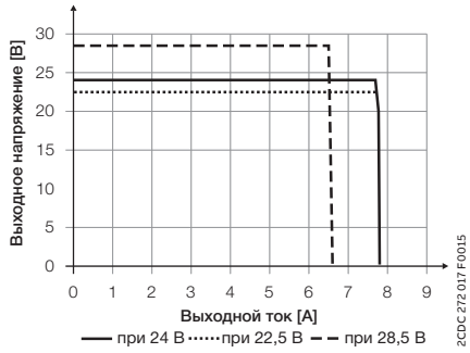
CP-C.1 24/5.0
