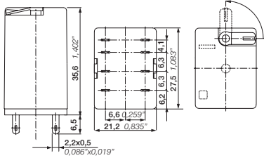
Реле CR-M с 2 переключающими контактами
