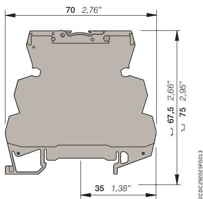
Исполнения с винтовыми клеммами
