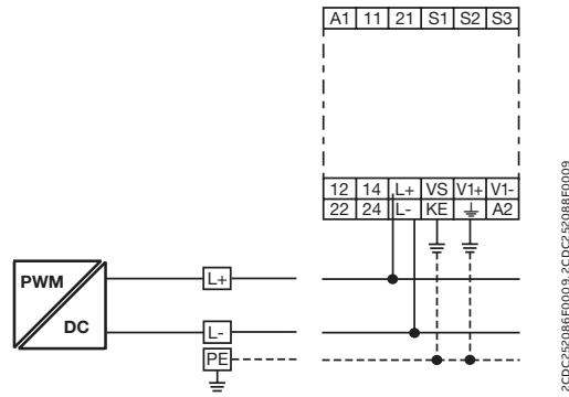
2-проводная сеть постоянного тока
