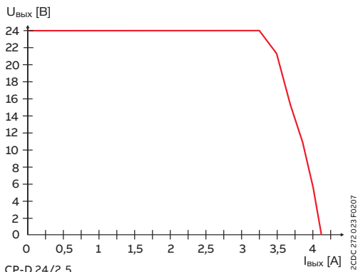
CP-D 24/2.5
