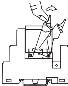
Демонтаж
