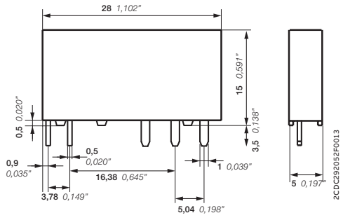
Реле CR-S
