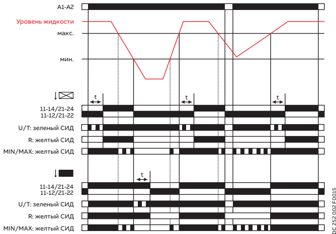
Слив: CM-ENS.31
