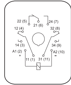
CR-U с 3 переключающими контактами
