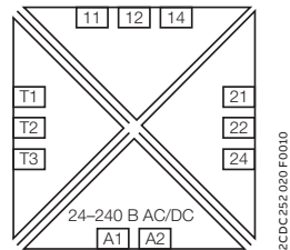
CM-TCS.1x
