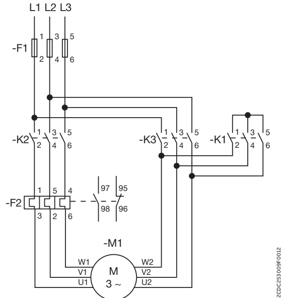
Схема силовой цепи
