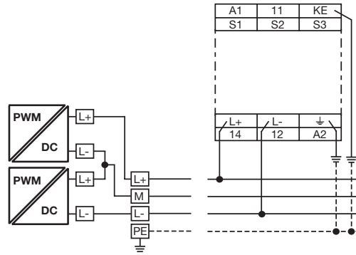
3-проводная сеть постоянного тока
