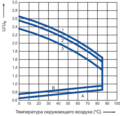
Диапазон рабочего напряжения и температуры катушки постоянного тока
