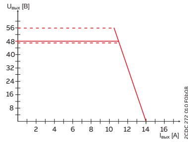
CP-E 48/10.0
