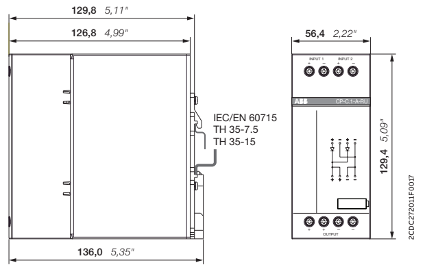
CP-C.1-A-RU
