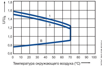
Диапазон рабочего напряжения и температуры катушки переменного тока
