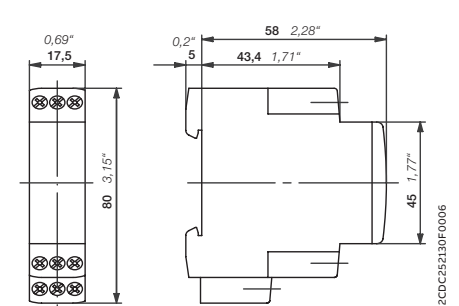
Устройства СТ-D с 2 переключающими контактами
