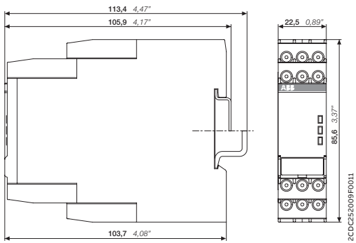
Основное устройство
