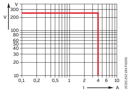
Нагрузка АС (резистивная)
