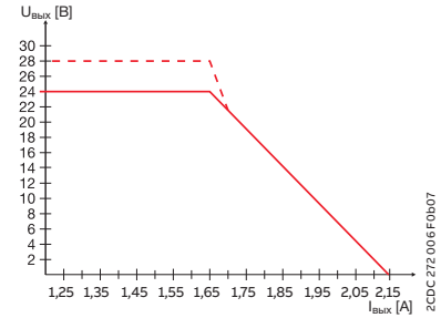
CP-E 24/1.25
