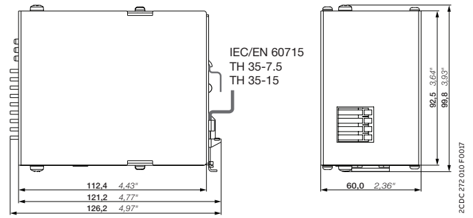
CP-B EXT.2
