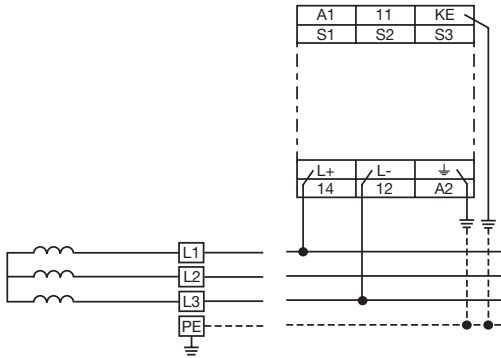
3-проводная сеть переменного тока
