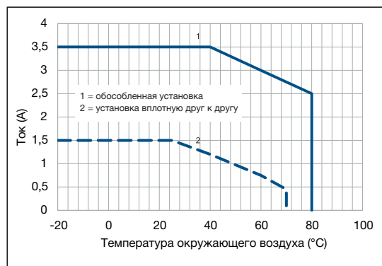
Выход CR-P с симистором
