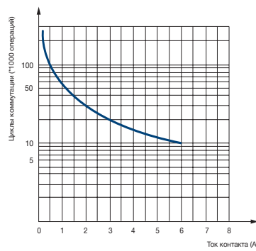
Кривая износоустойкости
