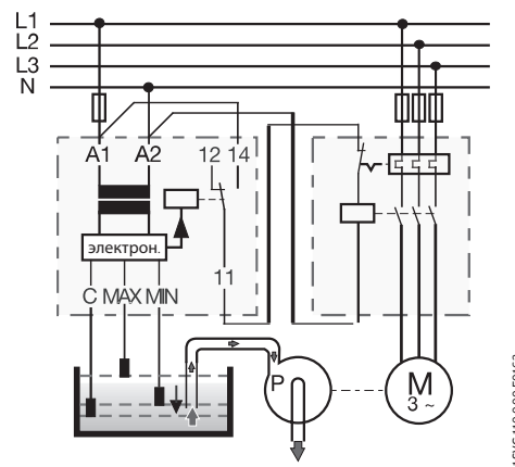
Контроль уровня жидкости — слив: выбрана функция ↓ (DOWN)
