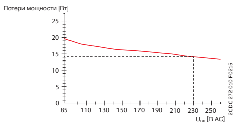
График зависимости средних потерь мощности (тепловыделения) от входного напряжения переменного тока
