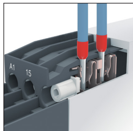
01 Монтаж проводников без инструментов
