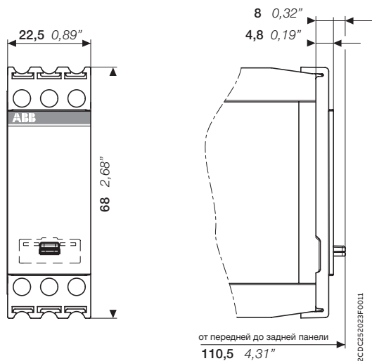
Пломбируемая крышка COV:11
