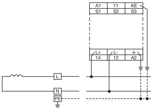
2-проводная сеть переменного тока
