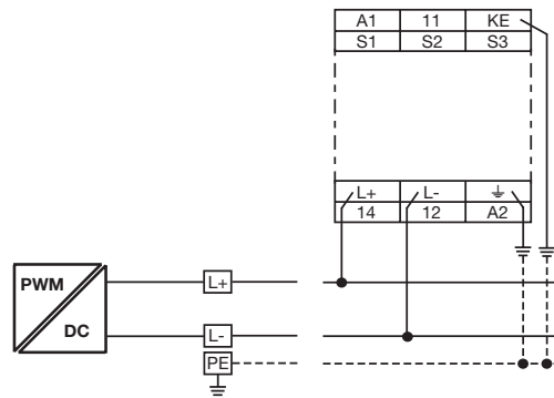
2-проводная сеть постоянного тока
