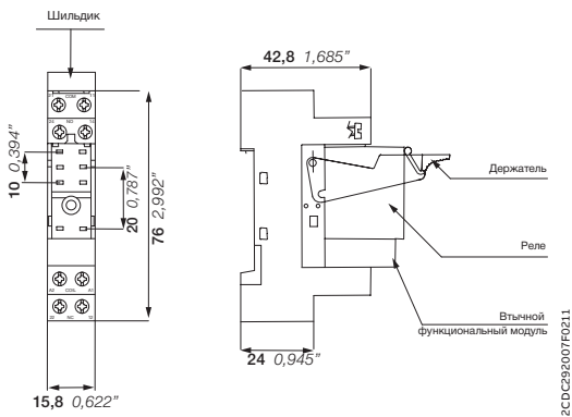
CR-PSS с винтовыми клеммами
