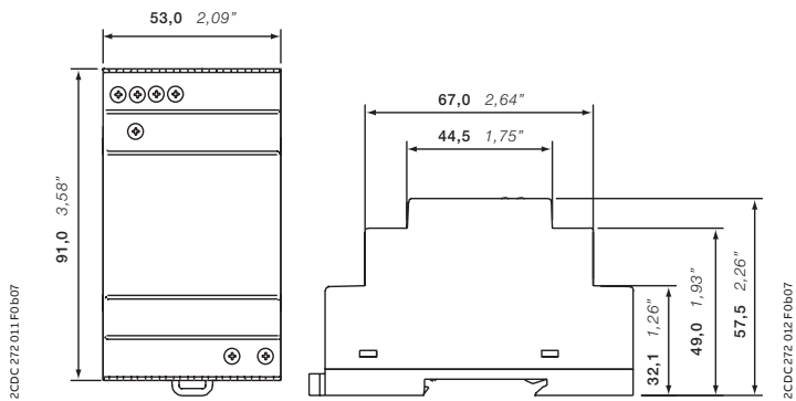
CP-D 12/2.1, CP-D 24/1.3
