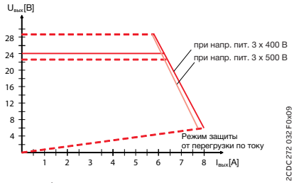
CP-T 24/5.0
