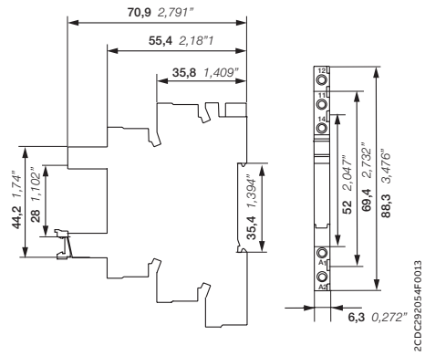
Цоколь CR-S с винтовыми клеммами
