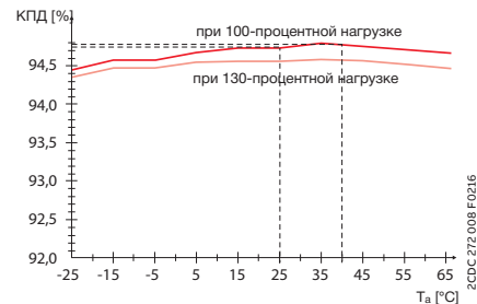
График зависимости среднего КПД от температуры окружающей среды
