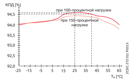
График зависимости среднего КПД от температуры окружающего воздуха
