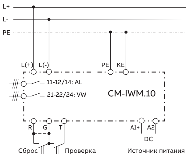
Пример использования в сети постоянного тока
