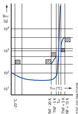
Характеристики термисторного датчика (РТС)
