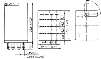
Реле CR-M с 4 переключающими контактами
