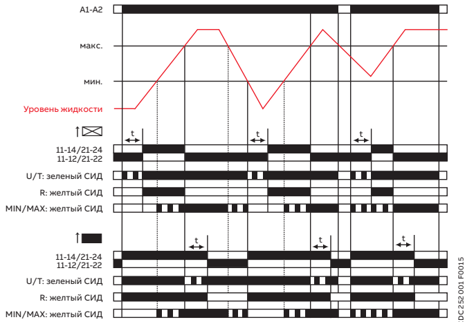
Наполнение: CM-ENS.31
