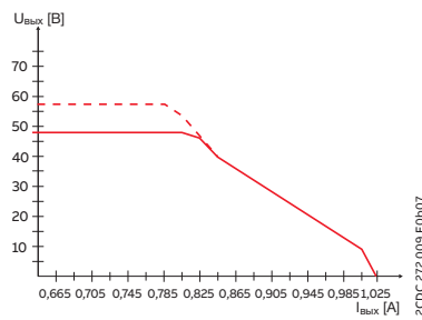
CP-E 48/0.62
