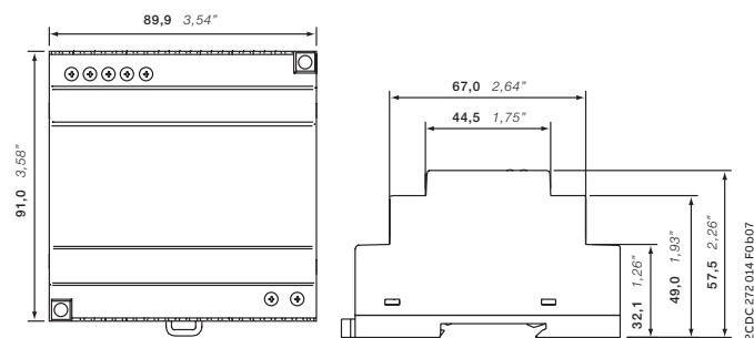
CP-D 24/4.2
