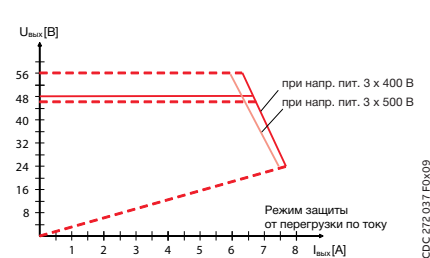
CP-T 48/5.0
