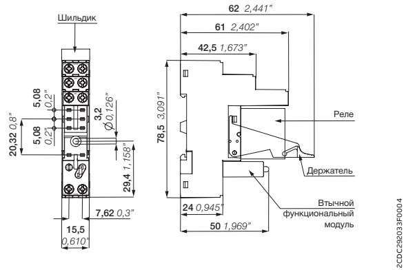
CR-PLSx с винтовыми клеммами
