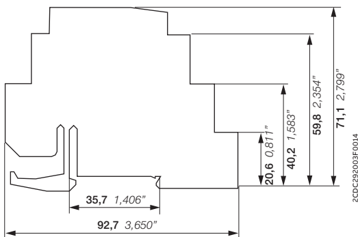
Разделитель CR-S
