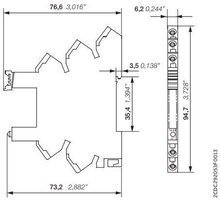
Цоколь CR-S с пружинными клеммами
