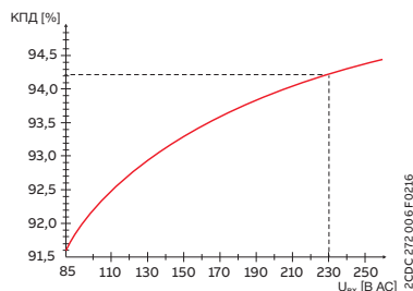
График зависимости среднего КПД от входного напряжения переменного тока
