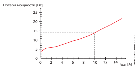
График зависимости средних потерь мощности (тепловыделения) от выходного тока
