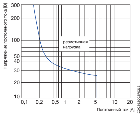
Исполнения с 1 НО, 1 НЗ или 1 переключающим контактом
