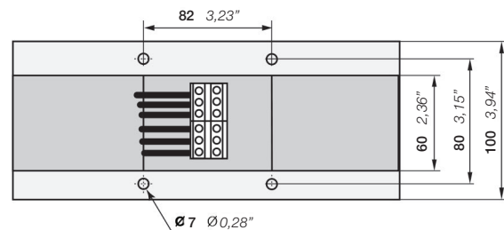
CT5L500R/4, CT5L850R/4
