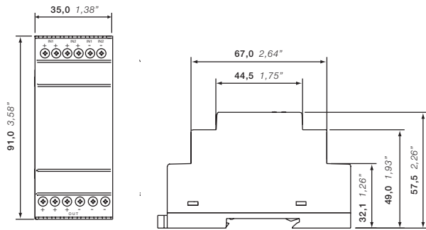
CP-D RU
