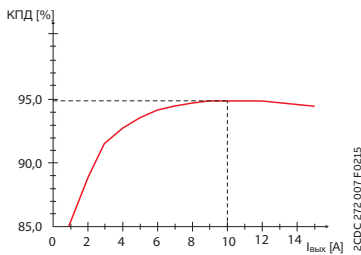
График зависимости среднего КПД от выходного тока
