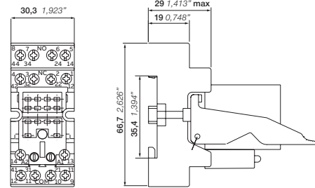
CR-MxSF с винтовыми клеммами
