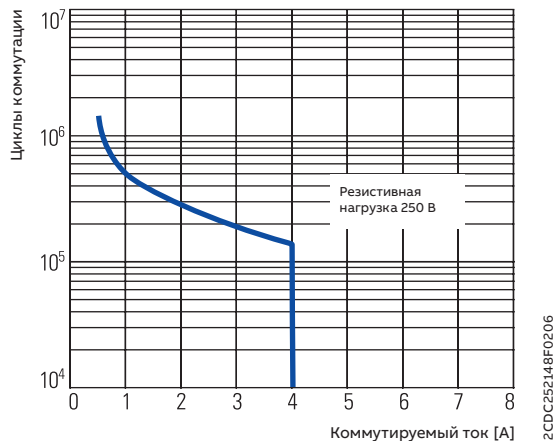
Срок службы контактов
