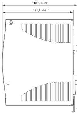
CP-T 24/5.0
