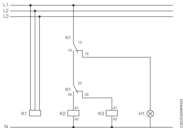
Схема цепи управления (K1 = CM-MPS.43 или CM-MPN.xx)
