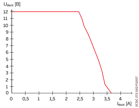
CP-D 12/2.1
