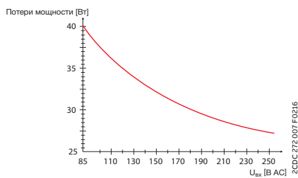
График зависимости средних потерь мощности (тепловыделения) от входного напряжения переменного тока
