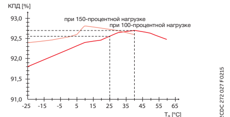
График зависимости среднего КПД от температуры окружающего воздуха
