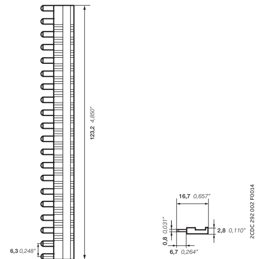
CR-SJB20 — синяя перемычка, CR-SJB20 — красная перемычка, CR-SJB20 — черная перемычка
