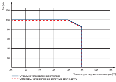
Транзисторный выход CR-S
