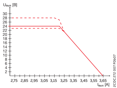
CP-E 24/2.5
