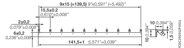
Перемычка CR-PJ
