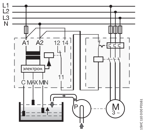
Контроль уровня жидкости — наполнение: выбрана функция ↑ (UP)
