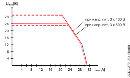
CP-T 24/20.0 Режим снижения напряжения при перегрузке
