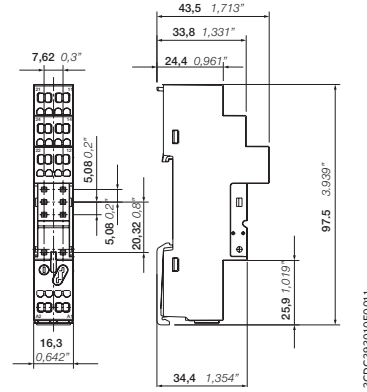
CR-PLS с пружинными клеммами
