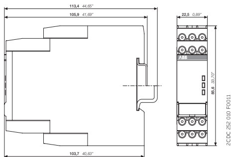
Серия СМ-S
