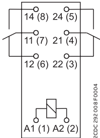
CR-P с 2 переключающими контактами
