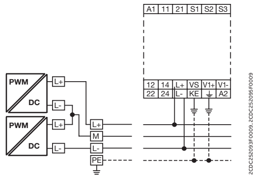
3-проводная сеть постоянного тока
