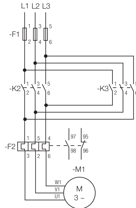
Схема силовой цепи
