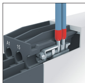
02 Подключение проводников к двойным винтовым клеммам с помощью отвертки
