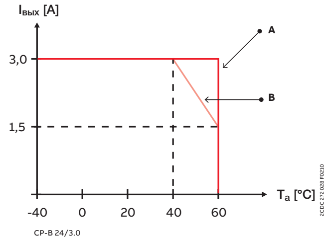
Температурные кривые при номинальной нагрузке
