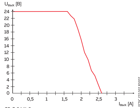
CP-D 24/1.3
