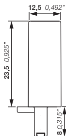
Функциональный модуль CR-P/Mxx
