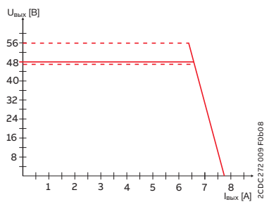
CP-E 48/5.0
