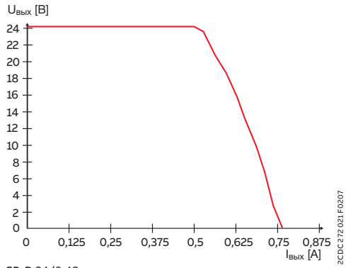
CP-D 24/0.42
