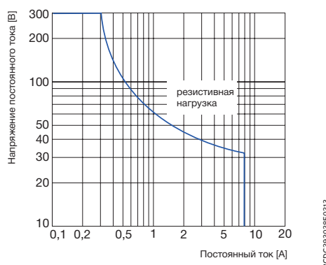
Исполнения с 2 переключающими контактами
