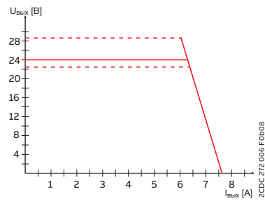
CP-E 24/5.0
