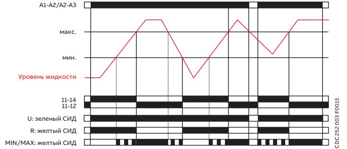
Наполнение: CM-ENS.2x
