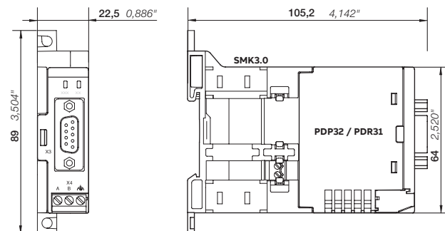
PDP32.0, PDR31.0
