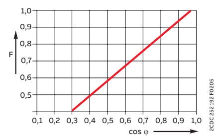
Коэффициент снижения F для индуктивной нагрузки АС
