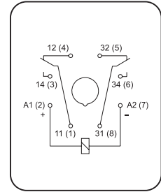
CR-U с 2 переключающими контактами
