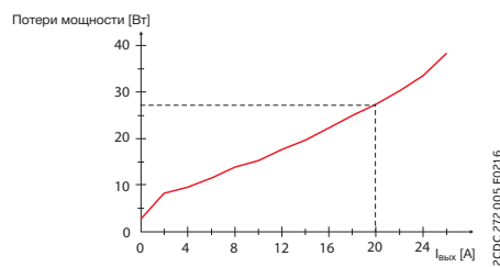
График зависимости средних потерь мощности (тепловыделения) от выходного тока
