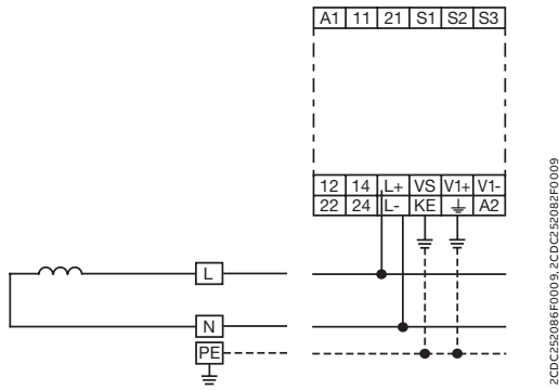
2-проводная сеть переменного тока
