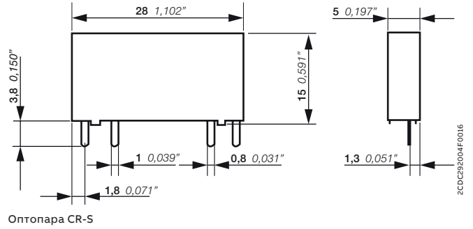
Оптопара CR-S
