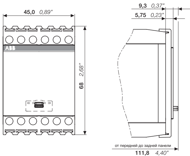
Пломбируемая крышка COV:12
