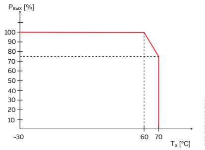
CP-T 24/20.0, CP-T 48/10.0
