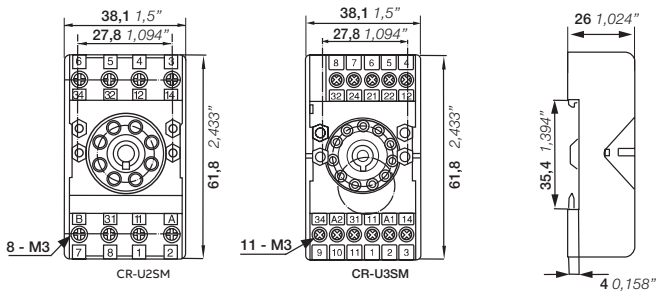
CR-U2SM — CR-U3SM с винтовыми клеммами
