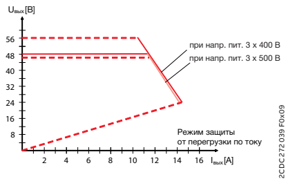
CP-T 48/10.0 Режим прерывания питания (hiccup mode) при перегрузке
