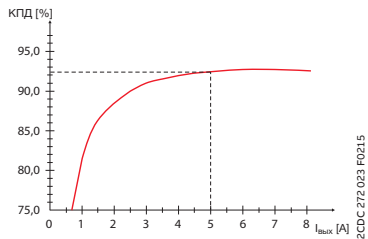
График зависимости среднего КПД от выходного тока
