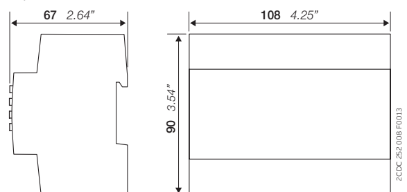
Серия СМ-UFD
