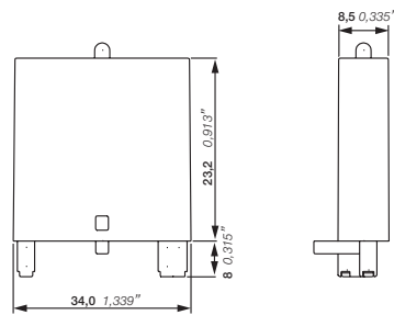
Функциональный модуль CR-Uxx
