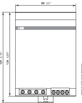
CP-T 24/10.0, CP-T 48/5.0
