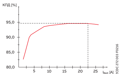
График зависимости среднего КПД от выходного тока
