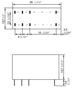
Реле CR-P
