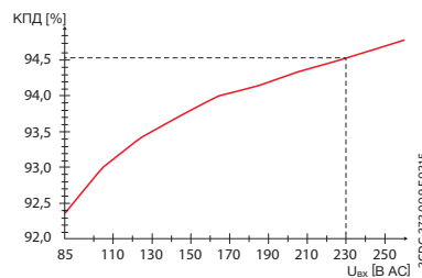
График зависимости среднего КПД от входного напряжения переменного тока
