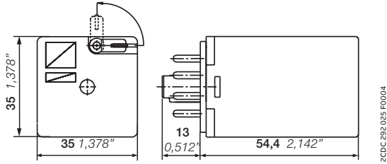
Реле CR-U с 2 переключающими контактами
