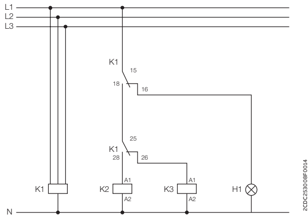
Схема цепи управления (K1 = CM-MPS.23)
