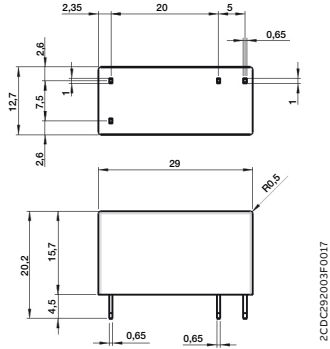
Оптопара CR-P
