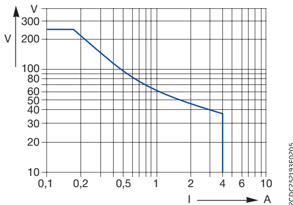
Нагрузка DC (резистивная)
