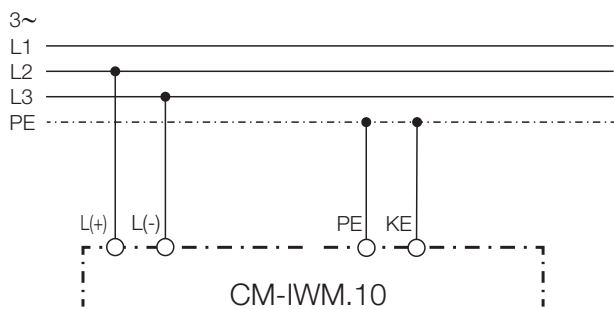
Пример использования в сети переменного тока
