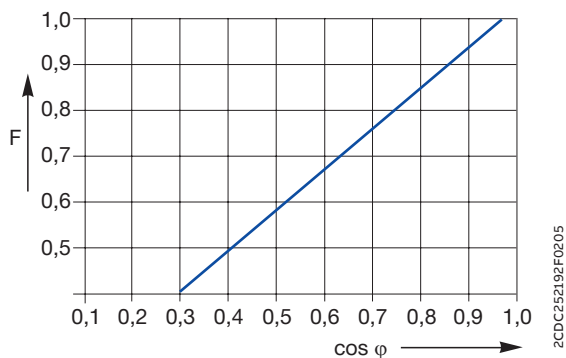
Коэффициент снижения F для индуктивной нагрузки AC
