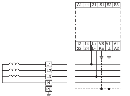
4-проводная сеть переменного тока
