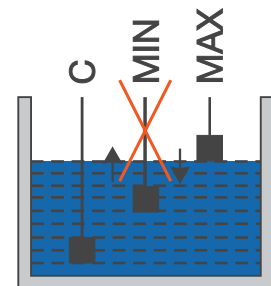
Режим работы с двумя электродами
