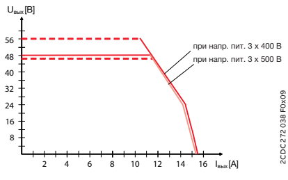
CP-T 48/10.0 Режим снижения напряжения при перегрузке
