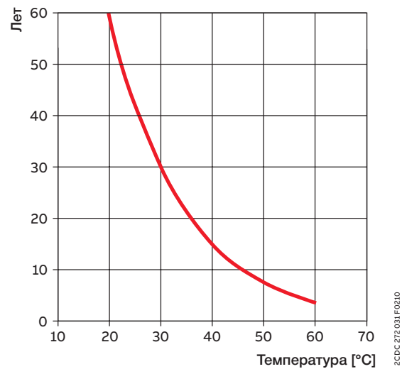
График зависимости срока службы конденсаторов от температуры
