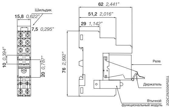
CR-PLS с винтовыми клеммами
