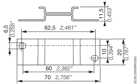
Адаптер для винтового крепежа ADP.01
